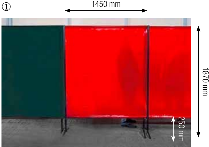
Abbildung zeigt mehrere Schutzwände aneinandergereiht
